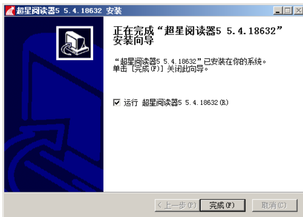
图 6 安装完成
