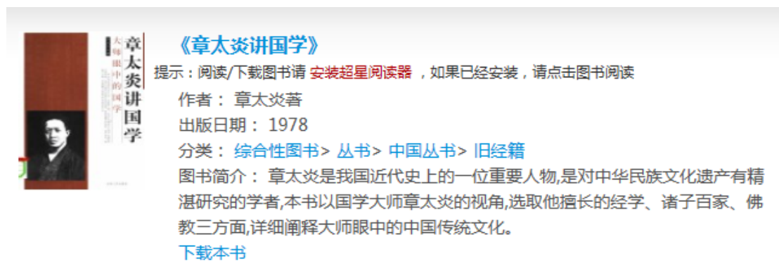
图 21 页面提示
