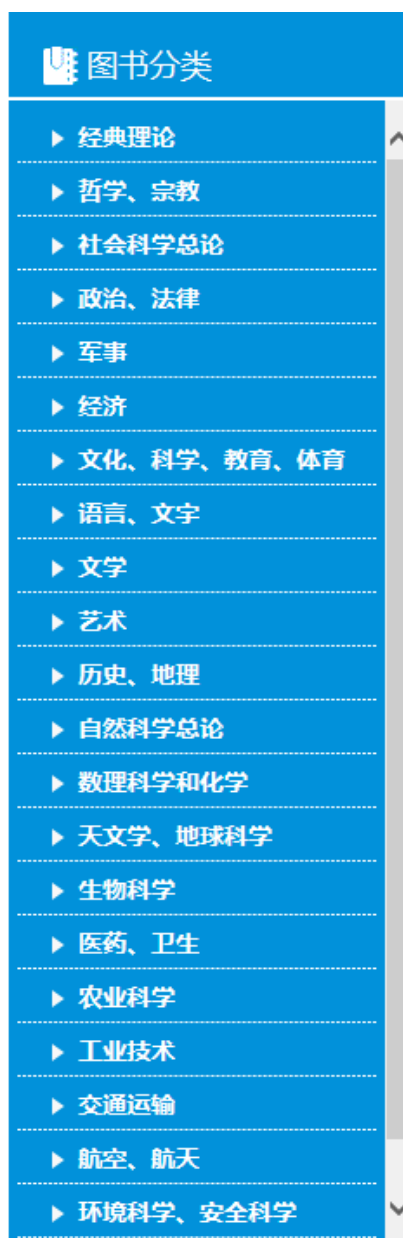
图 7 分类列表
