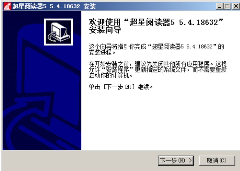
图 4 安装向导
