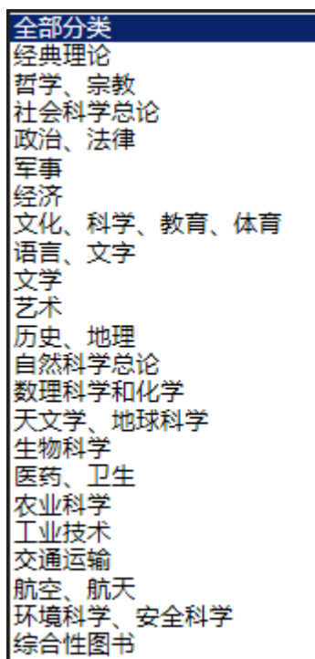
图 10 分类下拉框
